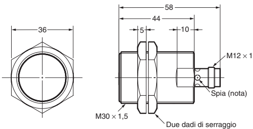
E2A-M30KS15-M1-□□/E2A-S30KS15-M1-□
