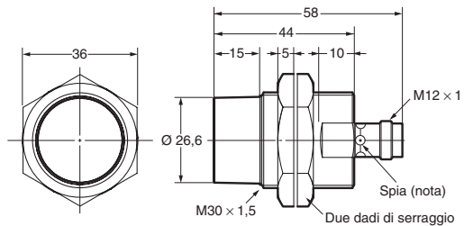
E2A-M30KN20-M1-□□/E2A-S30KN20-M1-□
